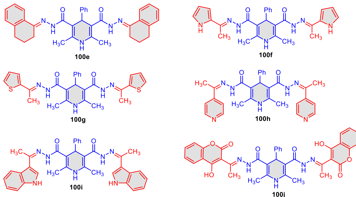
Scheme 22. Synthesis of bis -hydrazones 99a-f and 100a-j .
